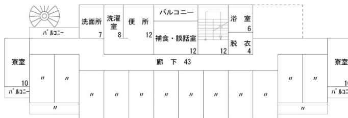
2～5階平面図→
