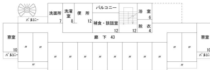
2～5階平面図→
