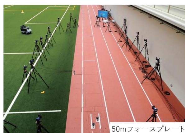
50m フォースプレート
